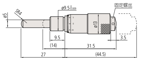
148-132 重量: 30g
