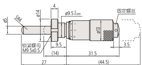
固定装置厚度: 6mm 重量: 35g 148-133
