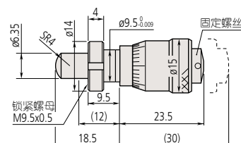
固定装置厚度: 6mm 重量: 35g 148-323
