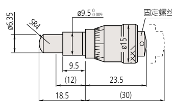
148-322 重量: 30g
